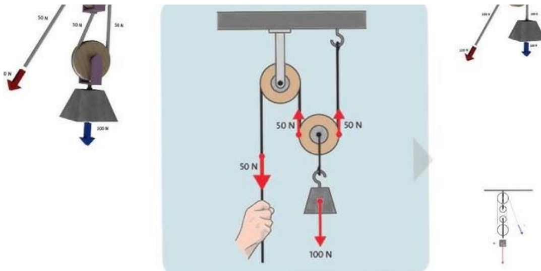
BRON 4 Met een kracht van 50 N kun je een gewicht van 100 N optillen.
